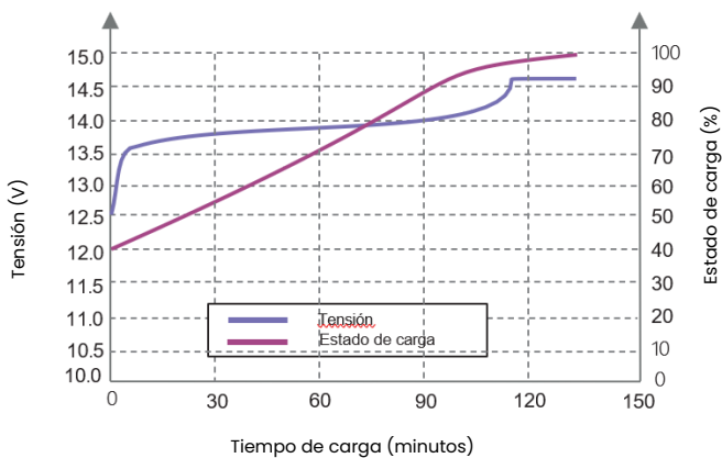
Curvas de estado de carga (0.5C, 25° C)
